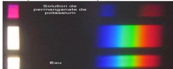
Spectre de bandes d'absorption de solutions
