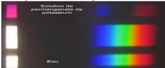
Spectre de bandes d'absorption de solutions
